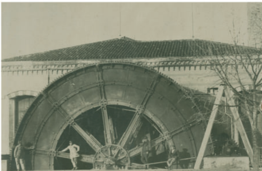
Fig. 3 - La ruota idrovora dell'impianto di Santa Margherita di Codevigo (1888)
