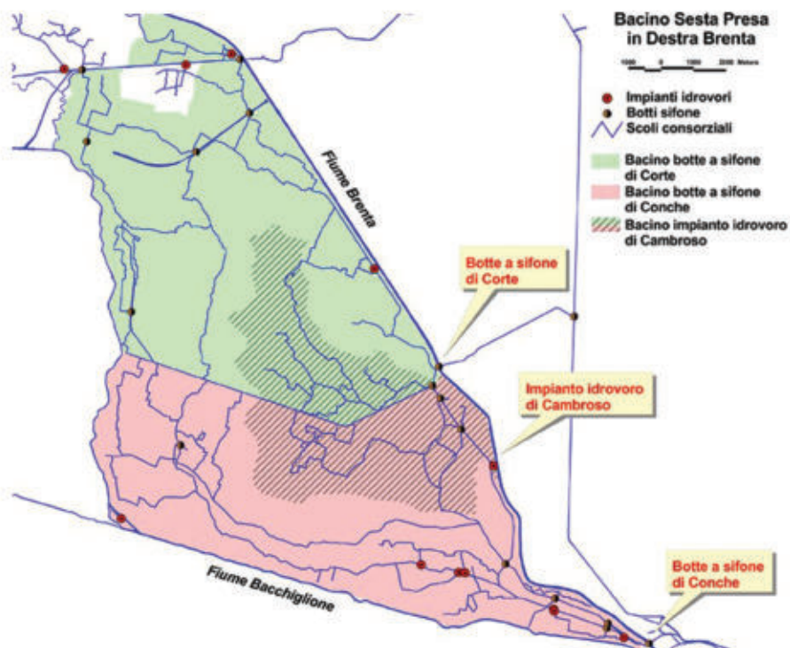
Fig. 8 - L'impianto idrovoro di Cambroso sottrae, nei momenti di piena, una parte della portata alle botti a sifone di Corte e di Conche
